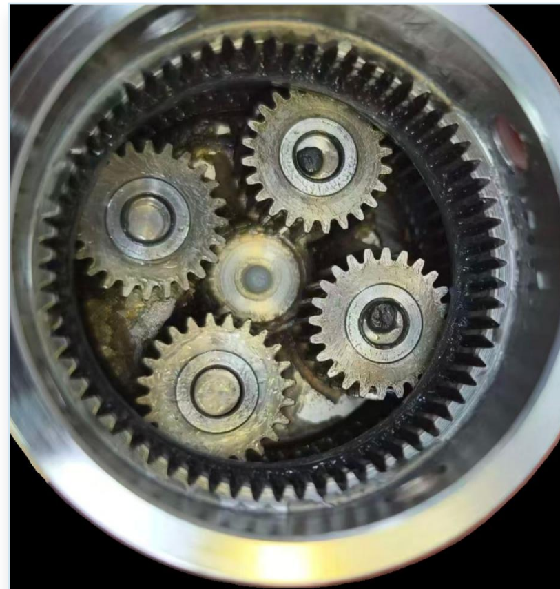
行星齿轮箱内部实况：多齿轮啮合、空间紧凑
